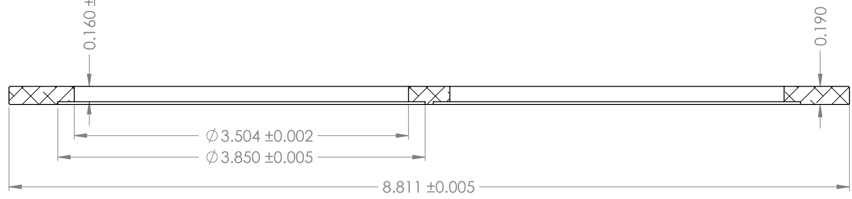
SECTION A-A
